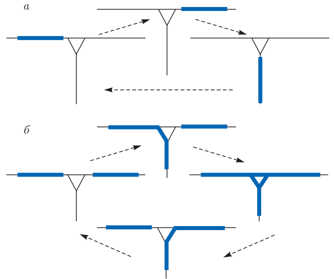
Рис. 2. Операция переплетения с ферромагнитными кубитами: а — однокубитное переплетение, б — двухкубитное переплетение. В процессе операций топологические области (жирные линии) сдвигаются из одной цепочки в другую, как показано на рис. Стрелками показан переход от одного этапа операции к следующему
