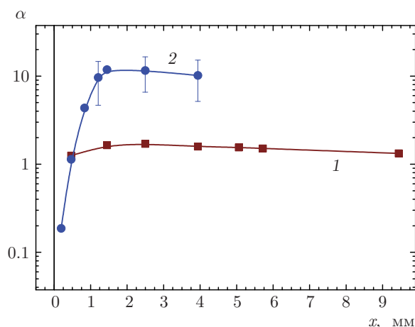
Рис. 6. Зависимости селективности \alpha диссоциации кластеров от расстояния зоны облучения частиц от сопла. Кривые 1 и 2 — степень разбавления соответственно 1/80 и 1/200. Мощность \text{CO}_2 -лазера 4 Вт, давление над соплом P_0 = 200 кПа
