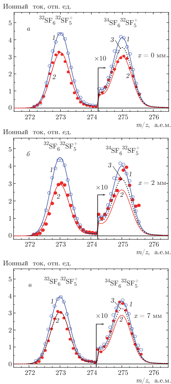
Рис. 4. (В цвете онлайн) Масс-спектры в области димерного ионного осколка \text{SF}_6\text{SF}_5^+ и его изотопных модификаций. Сплошные кружки — результат облучения. Синие кривые 1 — q = (1, 1, 1) . Красные кривые 2: а — q = (0.86, 0.86, 0.86) ; б — q = (0.83, 0.83, 0.83) ; в — q = (0.88, 0.88, 0.88) . Штриховые кривые 3: а — q = (0.86, 1, 1) ; б — q = (0.83, 1, 1) ; в — q = (0.88, 1, 1) (в области 273 а.е.м. кривые 3 совпадают с красными кривыми 2). \text{SF}_6/\text{Ar} = 1/200 ; P_0 = 163 кПа; мощность — 4.6 Вт (а), 4.8 Вт (б), 4.4 Вт (в); диаметр сопла — d = 0.16 мм. Расстояния от сопла: а — 0 мм (лазерный луч частично касается среза сопла); б — 2 мм; в — 7 мм
