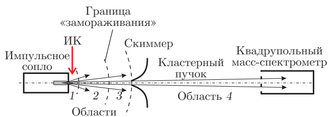
Рис. 1. Формирование кластерного пучка в условиях импульсной струи (подробнее см. текст)
