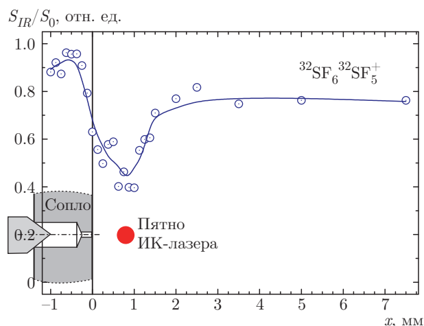
Рис. 3. Зависимость относительной величины кластерного сигнала S_{IR}/S_0 от положения лазерного луча (срез сопла и размер пятна лазера изображены на графике в масштабе). Струя облучалась на линии 10P(14) CO_2 -лазера (частота 949.48 см ^{-1} ), мощность излучения в камере 9 Вт. Над соплом использовалась смесь газов SF_6/Ar при соотношении давлений 1/100 и суммарном давлении P_0 = 133 кПа. Длительность импульса открывания сопла 1 мс (на полувысоте)
