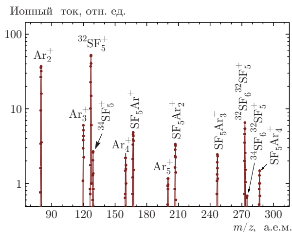
Рис. 2. Фрагмент масс-спектра продуктов ионизации кластерного пучка в диапазоне масс 70 \leq m/z \leq 300 а.е.м. Использовалась смесь \text{SF}_6/\text{Ar} при соотношении давлений 1/200, суммарное давление газа над соплом P_0 = 240 кПа
