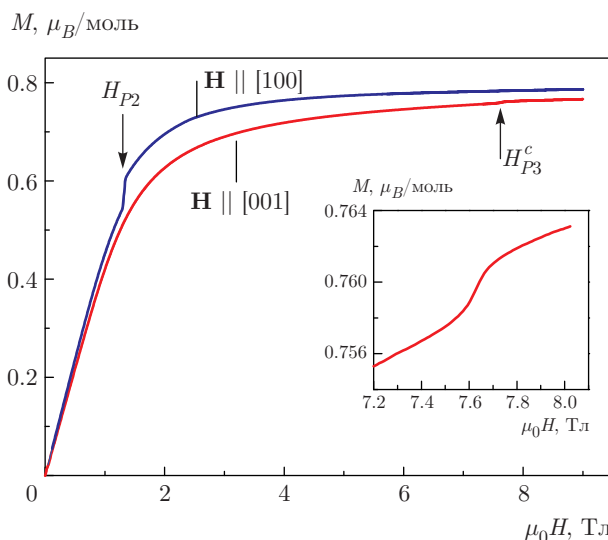
Рис. 4. (В цвете онлайн) Полевые зависимости магнитного момента при температуре 2 К. Магнитное поле направлено параллельно и перпендикулярно тетрагональной оси кристалла
