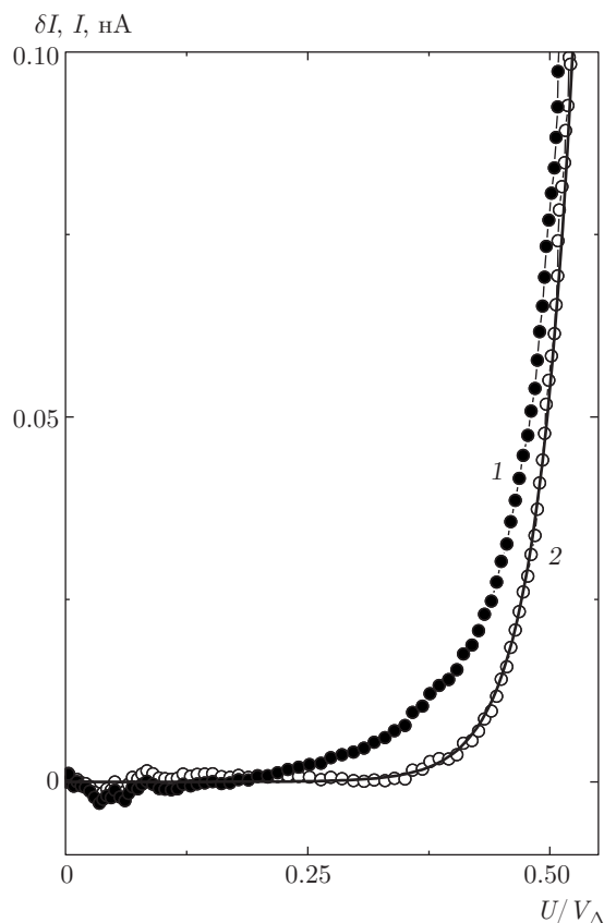
Рис. 5. Кружки — вольт-амперные характеристики для СИН-перехода за вычетом 1 — андреевского тока I_n , рассчитанного по формуле (3), и тока I_{Dy} по формуле (4); 2 — I_n + I_s , формула (3). Линия — одночастичный ток, формула (3), вычисленный при T = 0.085 К
