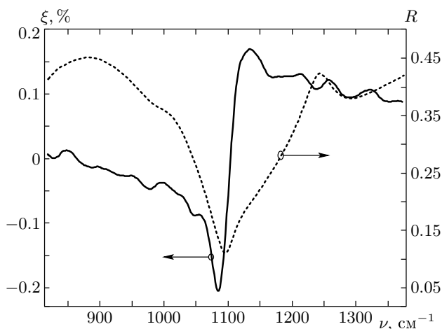
Рис. 5. Частотные зависимости коэффициента отражения (пунктир) пленки Fe-SiO 2 на подложке Si и магнитооптического эффекта (сплошная линия) для значения магнитного поля H = 2200 Э
