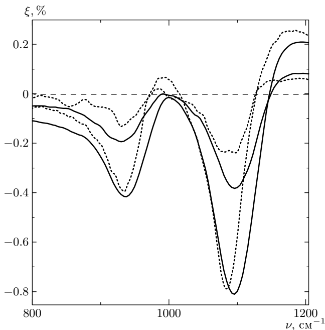
Рис. 6. Частотные зависимости магнитооптического эффекта пленки Co 43 Al 22 O 35 для двух значений поля \Delta H = 2200 Э, 100 Э: сплошные линии — для угла падения \varphi = 45^\circ ; пунктирные — \varphi = 10^\circ
