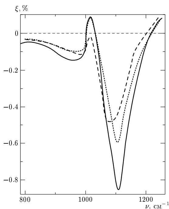
Рис. 7. Теоретические зависимости магнитооптического эффекта пленки Co 43 Al 22 O 35 : сплошная линия — \Delta\rho/\rho = 3\% , пунктир — \Delta\rho/\rho = 1\% (для \varphi = 45^\circ ); штриховая линия — \Delta\rho/\rho = 1\% , \varphi = 10^\circ
